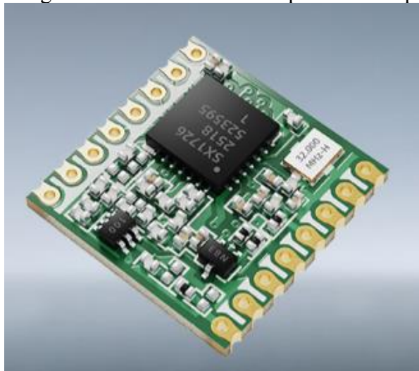
RFM95W
